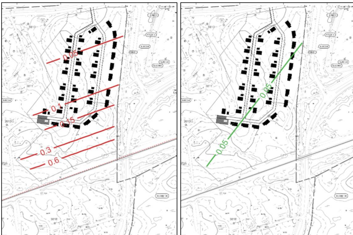
Kuvat 7 ja 8: Mallinnustulokset raideliikenteen aiheuttamasta tärinästä kaava-alueen massoitteiluonnoksella. Pohjoinen raide (kuva 7, vasemmalla) ja eteläinen raide (kuva 8, oikealla).
